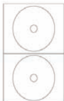
F.TO Ø 117,5 - FORO Ø 17 NR. 2 ETICHETTE PER CD LC235
